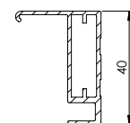
SECTION B-B (1 : 1)
